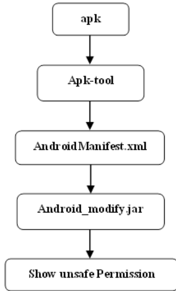
圖 6、Decompiler AndroidManifest
