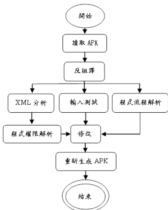
圖 5、系統架構
